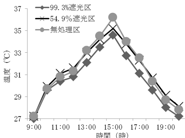
図－１ 果実袋の遮光率と果実温度
